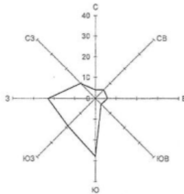
Рисунок 5.1 – Роза ветров
